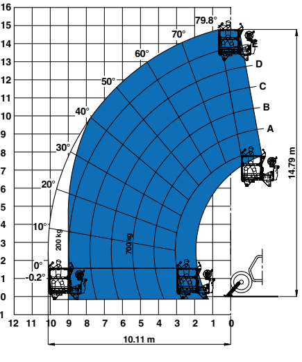
Sur stabilisateurs avec nacelle 3P-700REM 4400
