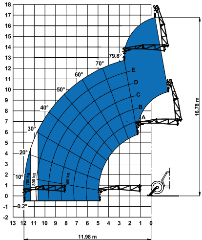
Sur stabilisateurs avec nacelle 3P-700REM 4400
